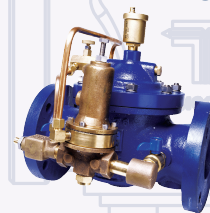
Válvula de Alivio Pilotada Serie VAP
